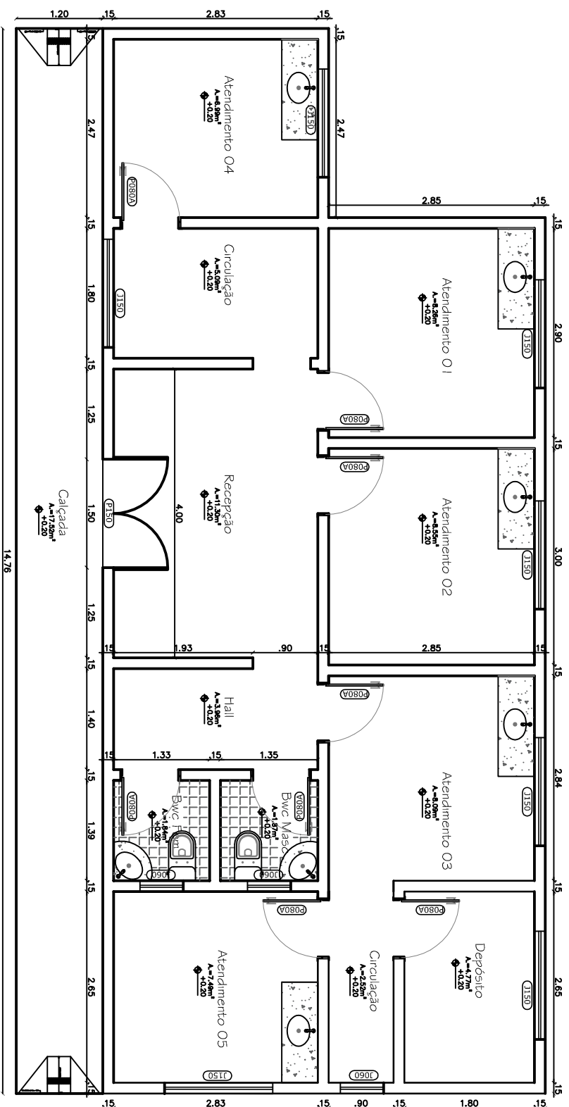
PLANTA BAIXA - Pav. Térreo ESCALA ..... 1:75 ÁREA CONSTRUÍDA ..... 82,69 m²
